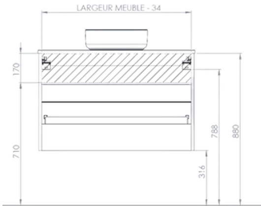
HAUTEUR D'INSTALLATION - INSTALLATION HEIGHT
