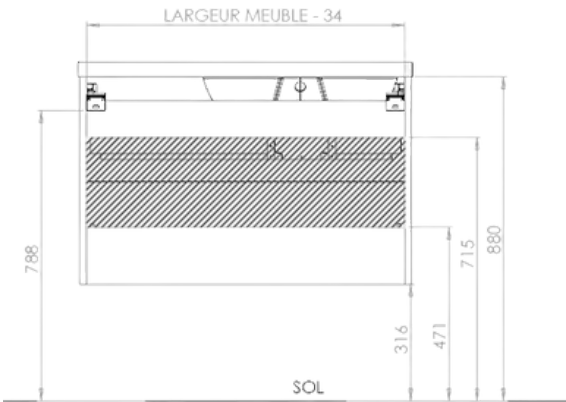
HAUTEUR D'INSTALLATION - INSTALLATION HEIGHT
