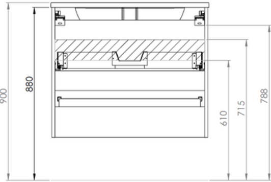
HAUTEUR D'INSTALLATION - INSTALLATION HEIGHT
