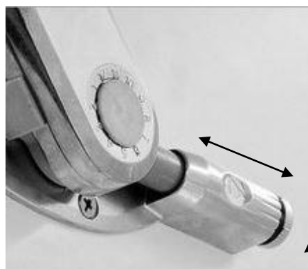
Tourner pour rentrer ou sortir l'amortisseur pour régler la puissance Screw or unscrew the damper to adjust the damping strength
