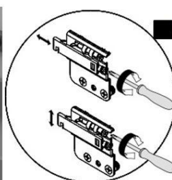
2 Serrer les accroche-meubles pour faire plaquer le meuble au mur et ajuster les niveaux Tighten the brackets on the unit so that the furniture fits to the wall and adjust the levels
